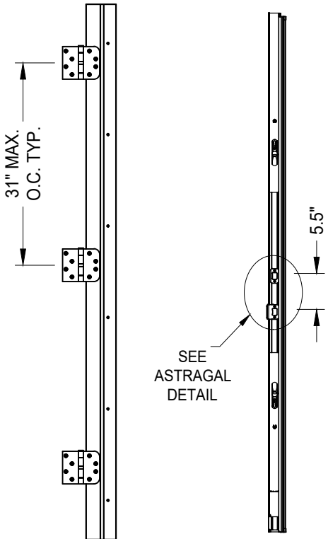
HINGE JAMB ASTRAGAL
