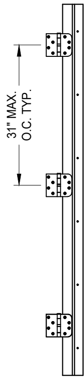
HINGE JAMB
